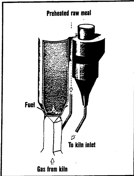
ILC-E calciner.
